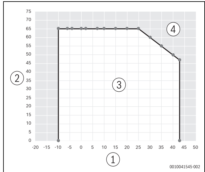
Bild 21 Betriebsart und Warmwasserbereitung in Abhängigkeit von der Umgebungslufttemperatur
